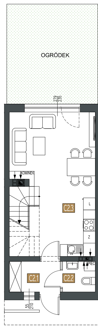
rzut parteru
