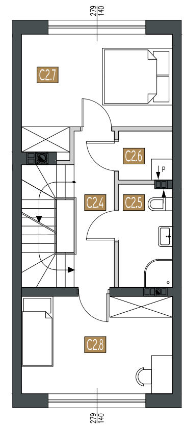
rzut 1 piętra
