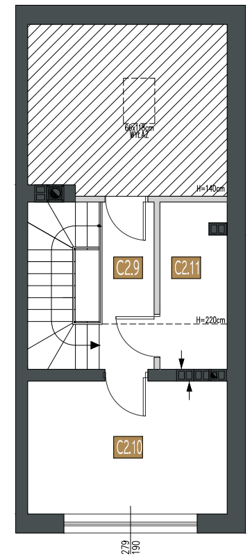
rzut strychu
