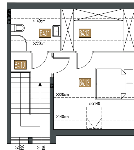
rzut strychu
