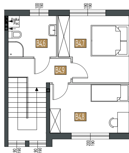
rzut 1 piętra
